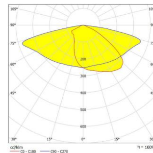
Distribuția Luminanței
